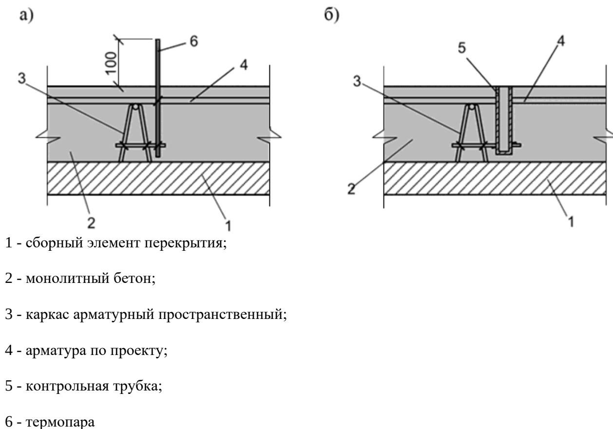
а) схема установки термопар; б) схема установки контрольных трубок
