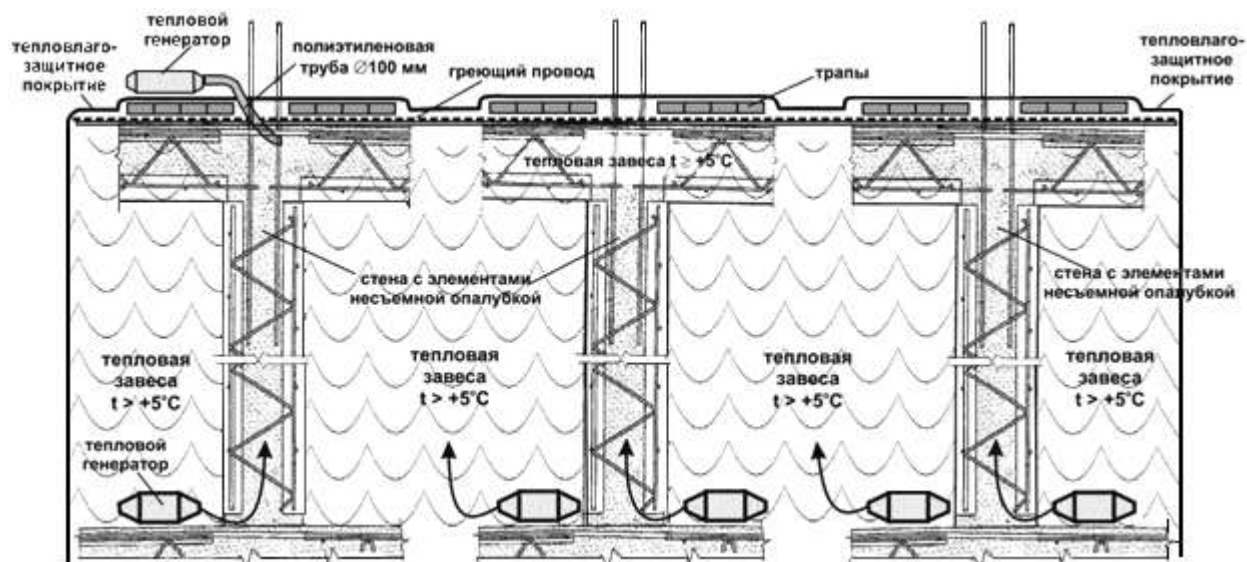
Рисунок 12 - Схема прогрева конструкций
