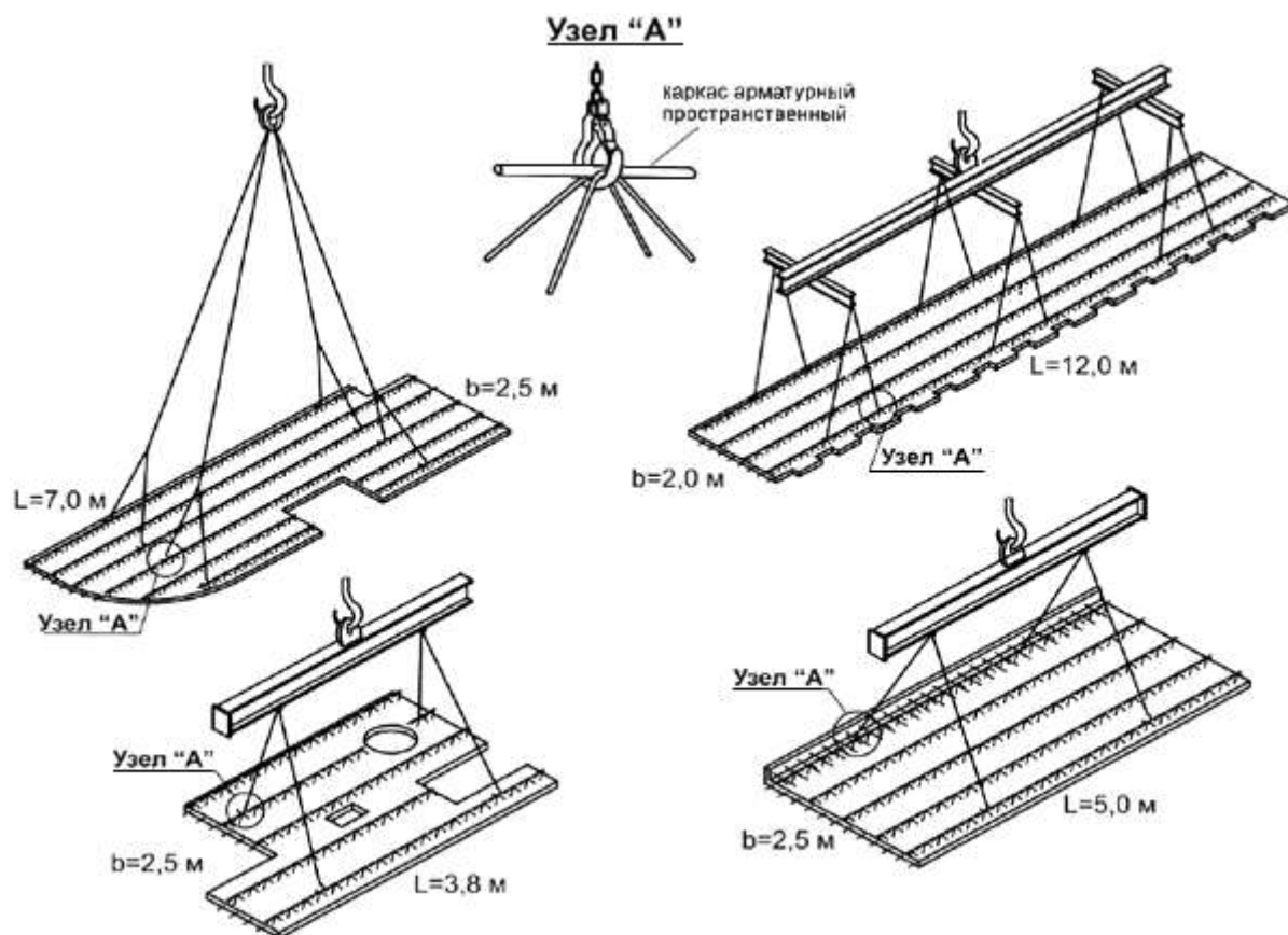
Рисунок Г.1 - Примеры строповок сборных элементов перекрытий
