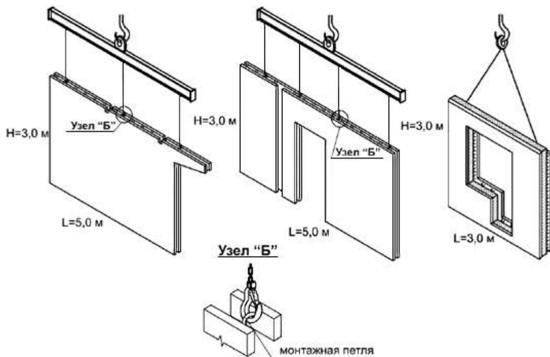
Рисунок Г.2 - Примеры строповок сборных элементов стен
